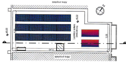
PIANTA PIANO COPERTURA
